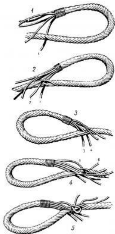
Рис. 7. Заделка огона на стальном тросе.
